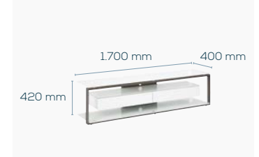
TV-Rack 5206
