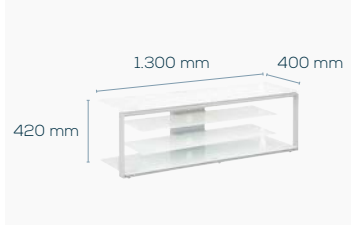
TV-Rack 5200
